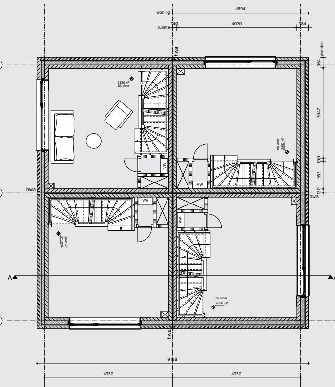
eerste verdieping
