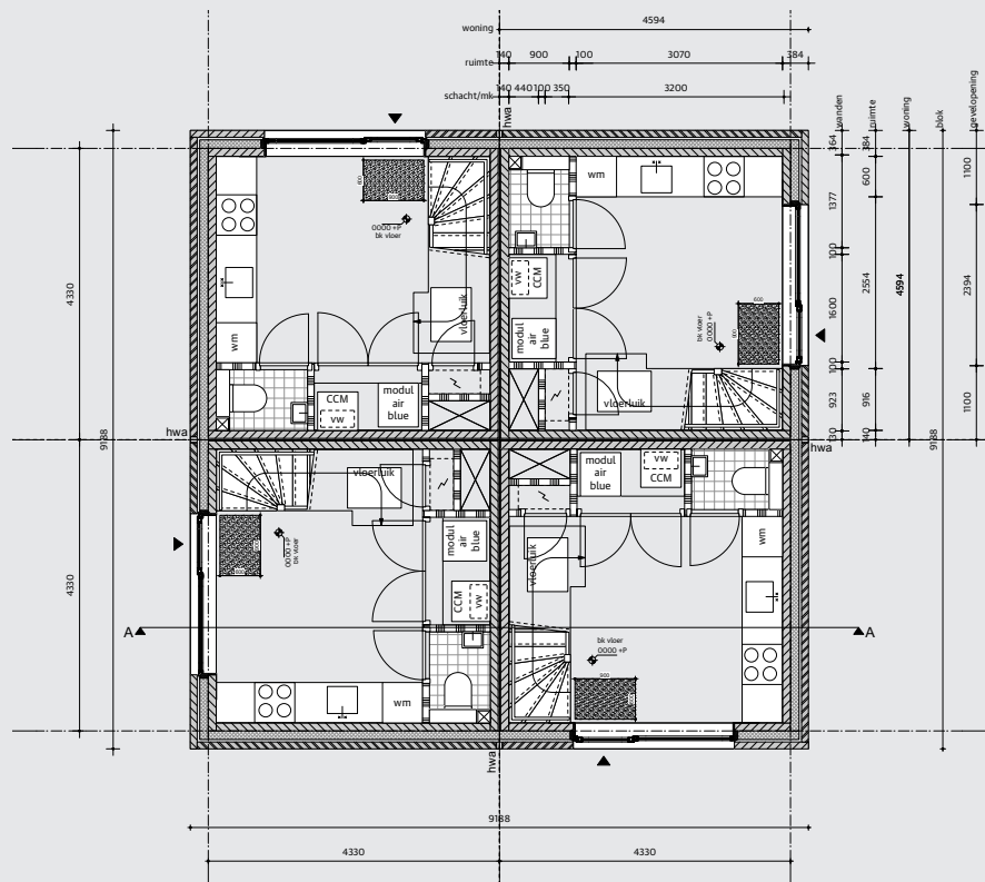
begane grond
