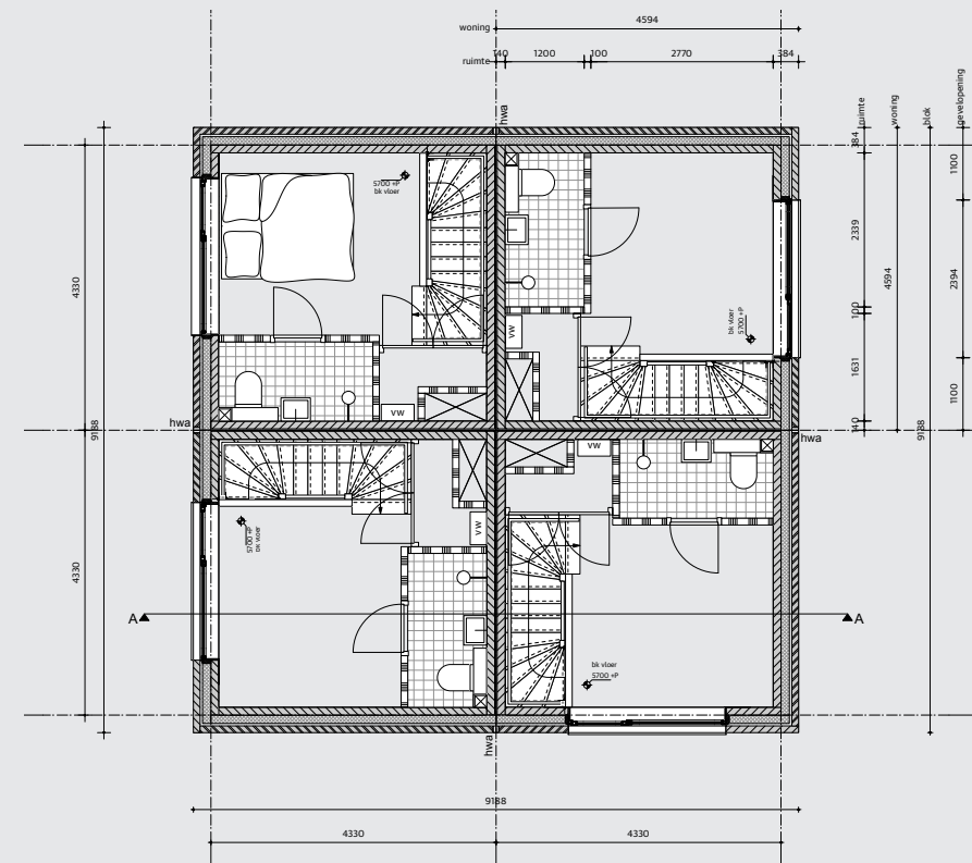
tweede verdieping
