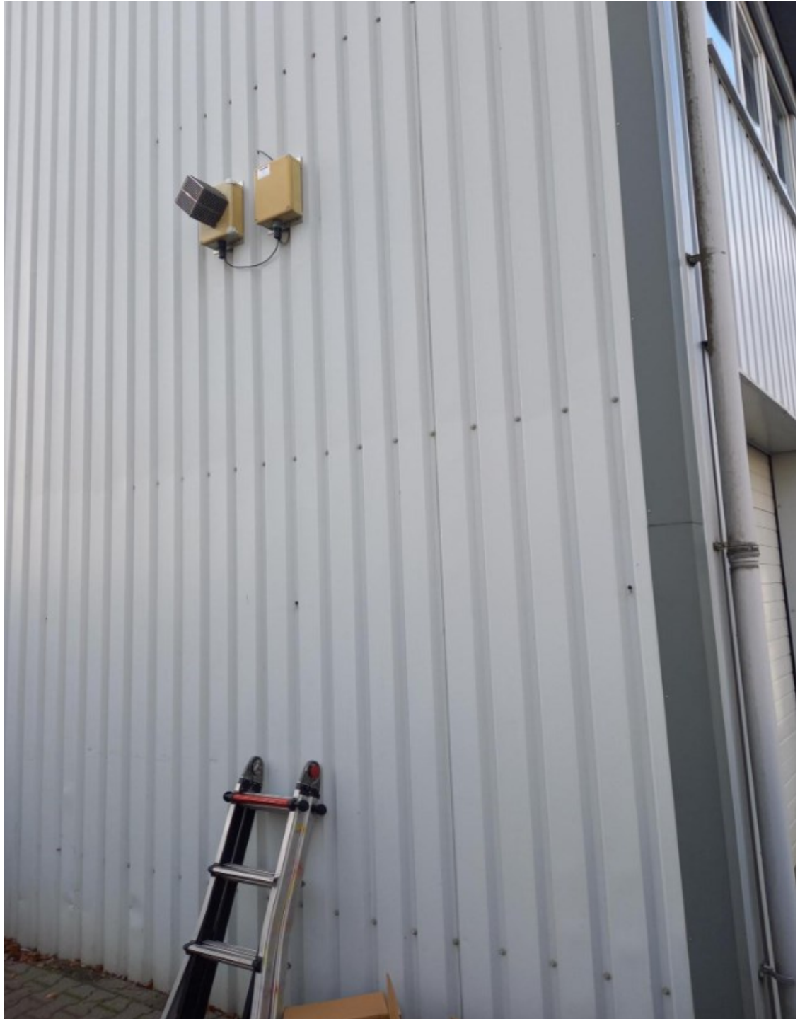
figuur 23: weergave meetopstelling
